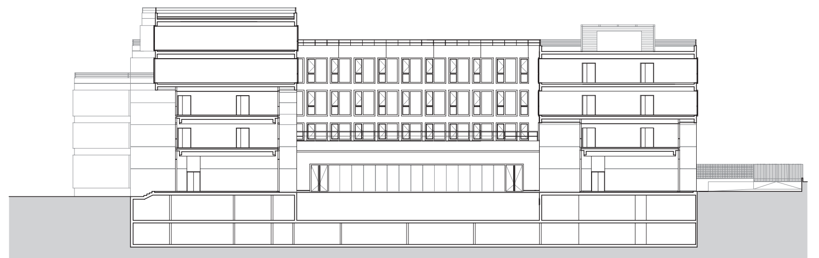
Elevation
